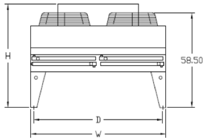
END VIEW FEV*25, FEV*26, FEV*27
